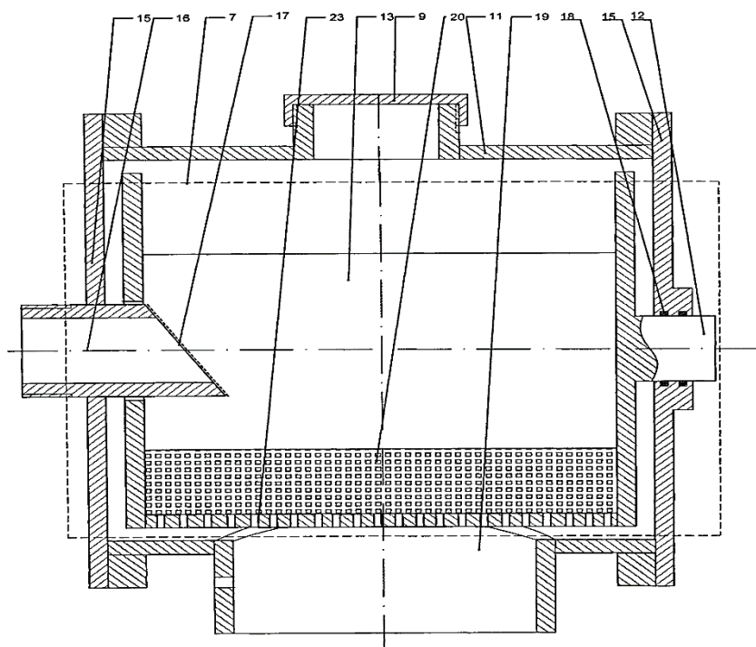
Рис. 1. Типовая конструкция аппарата с вращающимся электромагнитным полем [1,4]; 7 - дозатор; 9 - загрузочное устройство; 11 - камеру дозирования; 12 - приводной вал; 13 - поворотный бункер; 15 - крышка; 16 - патрубок промывки; 17 - скошенный торец; 18 - сальниковое устройство; 19 - выходной патрубок; 20 - сетка; 23 - перфорированное дно;
