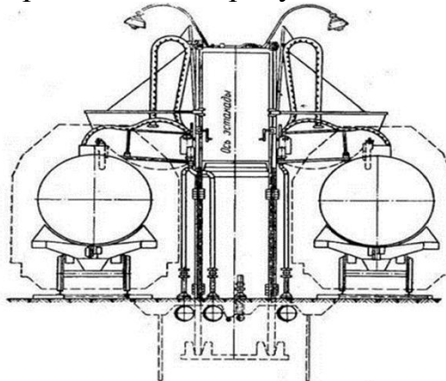
Рисунок 1. Общий вид эстакады
