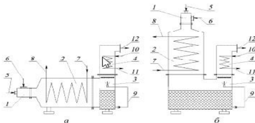
Рисунок 2 - Варианты расположения радиационной части.
