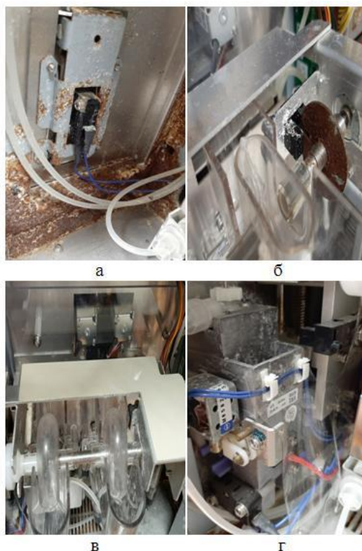
Рисунок 3. Фотографии узлов МЕК-6400 в процессе эксплуатации (а, б – следы коррозионного воздействия на оптических датчиках; в, г – пластиковые накладки для предотвращения попадания жидкости на датчики и двигатель).
