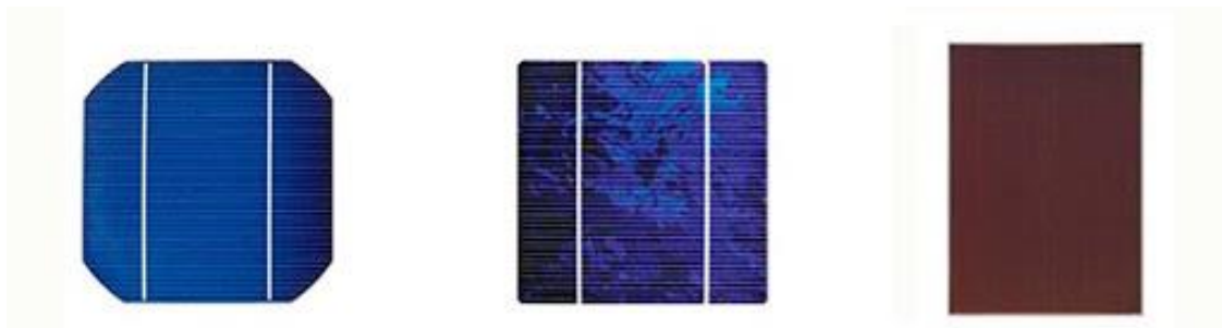
Рис. 1. Монокристаллический, поликристаллический и аморфный элементы.
