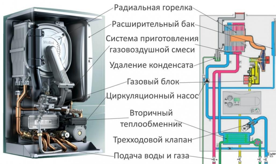
Рисунок 1 - Конструкция конденсационного газового котла.
