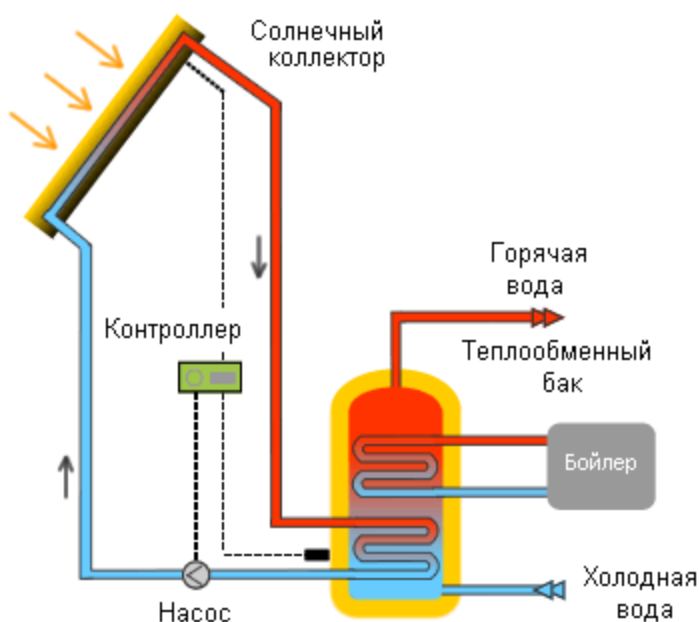
Рис. 2. Наглядное представление работы солнечного коллектора.
