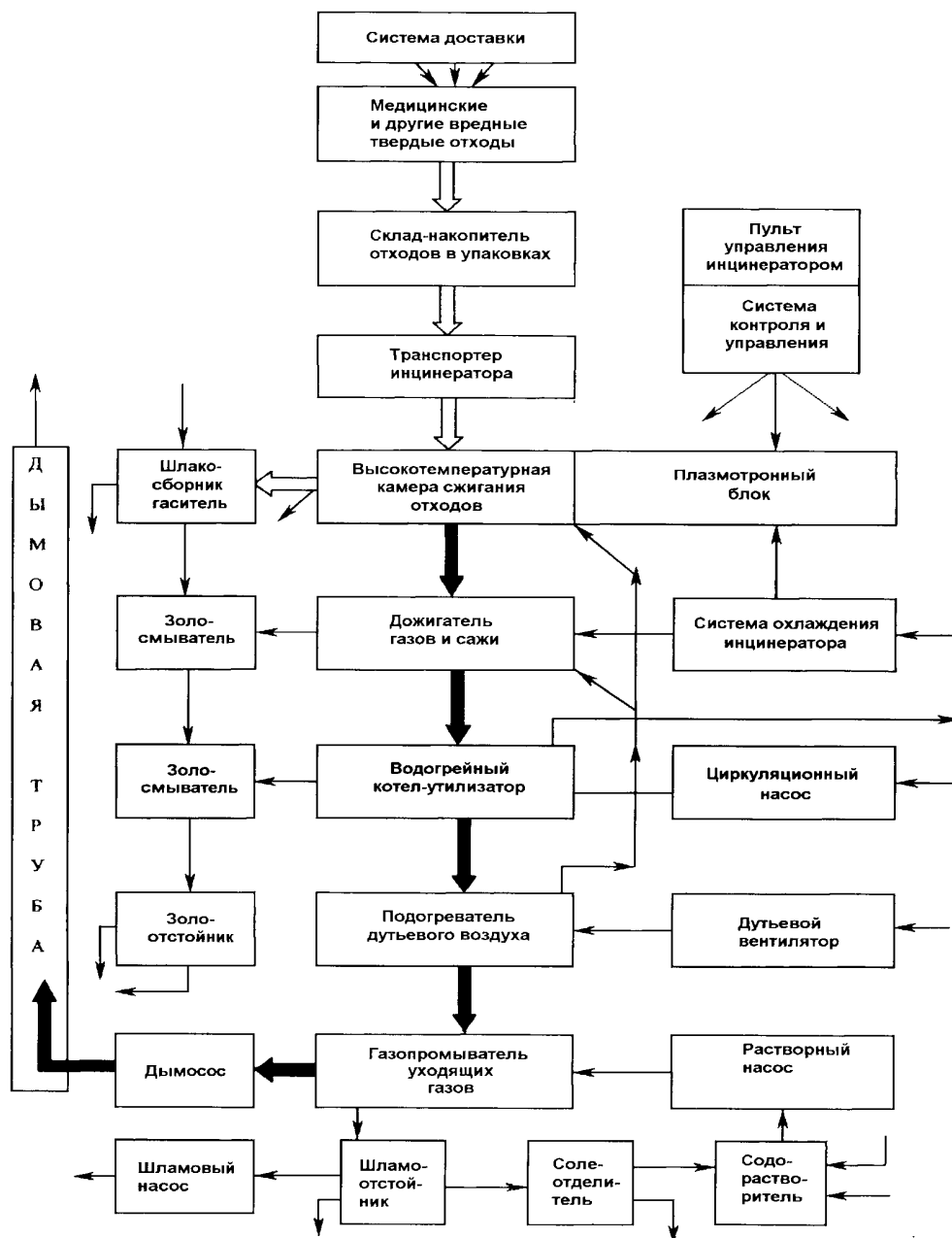
Рисунок 4. Блок-схема плазменной установки
